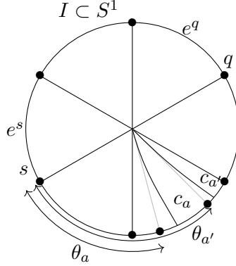
FIGURE 7.3. Les notations du cas \alpha_1 > \alpha_2 > \alpha_3 (dans la situation où s et q sont des sommets, et e^s, e^q sont de longueur exactement \pi/3 ).
