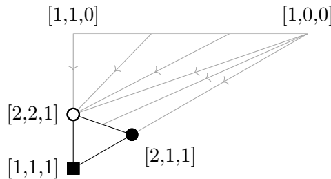
FIGURE 9.1. L'application \pi en restriction à une chambre de \mathbf{X}_3 .
