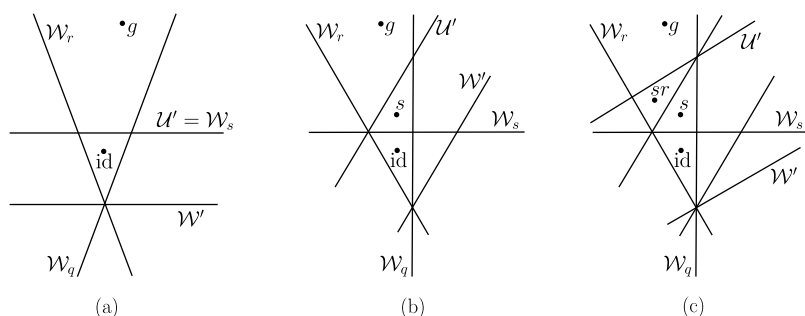
Fig. 1 Proof of Lemma 3.2
