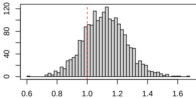
\Psi_0
