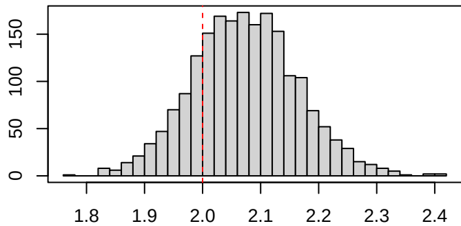
\Psi_2
