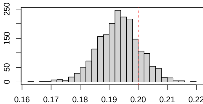
\Psi_1
