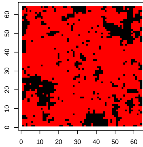
SW Iteration 20
